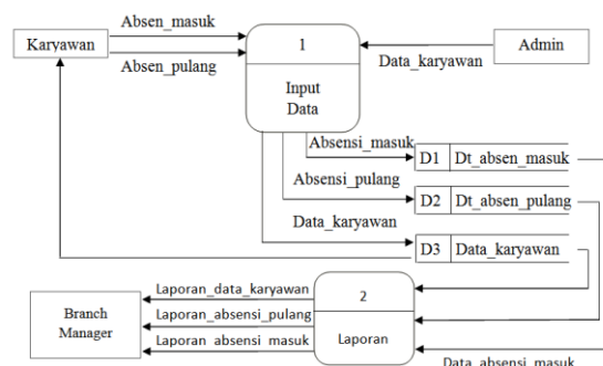
Gambar 2 DFD Level 0 Absensi Karyawan
