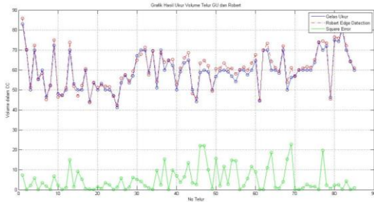
Gambar 11. Grafik SE antara GU dan Robert
