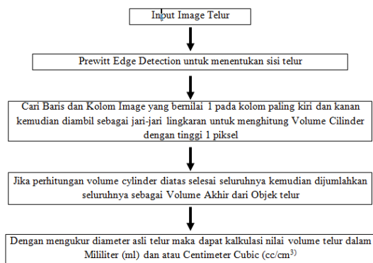
Gambar 2. Metode yang diusulkan
