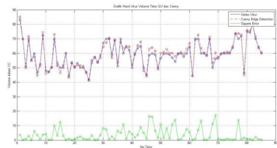
Gambar 10 Grafik SE antara GU dan Canny
