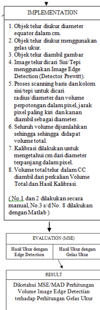
Gambar 1: Kerangka pemikiran
