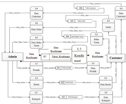
Gambar 4. DFD Level1
